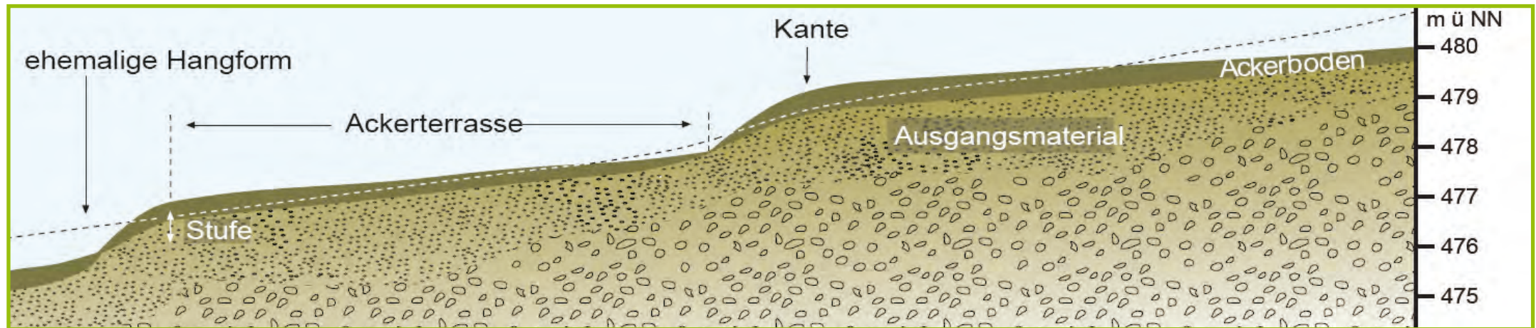
Schematische Darstellung der Entstehung von Ackerterrassen
