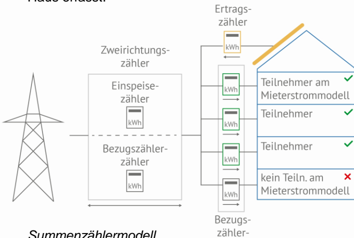
Summenzählermodell, Abb. Energieagentur Regio Freiburg GmbH
