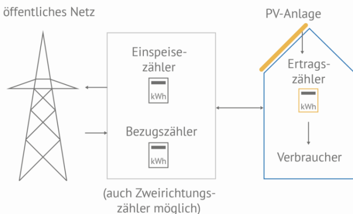
Bezugs-, Ertrags- und Einspeisezähler, Abb. Energieagentur Regio Freiburg GmbH
